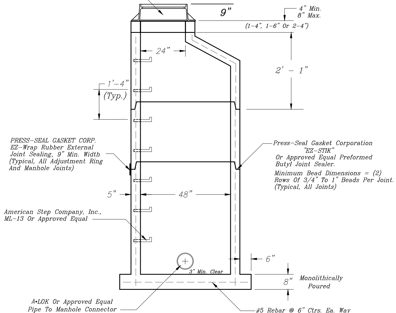
MANHOLE SECTION A Scale: 1" = 30"
